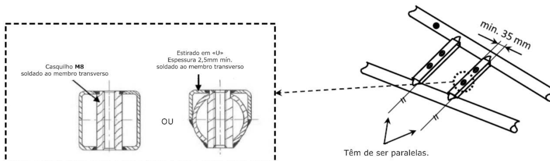
Figura 5 - Construção "C"
