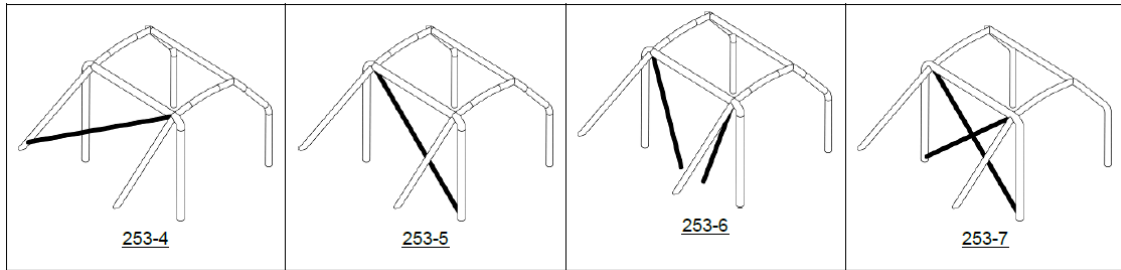
Figura 28 - Tipos de diagonais aceites - Anexo J - 253-4/5/6/7
