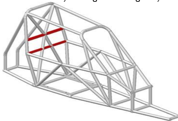
Figura 9 - Reforço transversal
